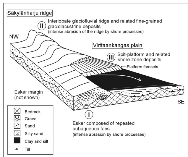
Figure 3 The structural zones of the Säkylänharju-Virttaankangas complex.
